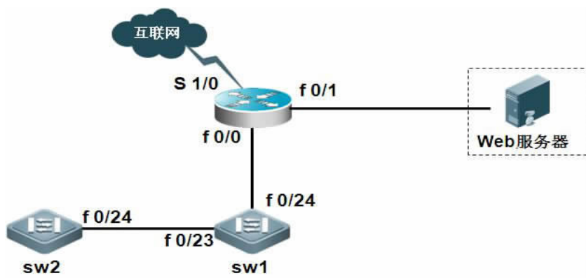
图 3-1 网络拓扑图
